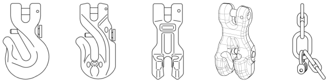
Verkortings- haken TWN 0827/1 TWN 0827 Verkortings- haken TWN 1827/1 TWN 1827 Verkortings- klauwen TWN 0851 TWN 1851 Verkortings- klauwen TWN 0851/1 TWN 1851/1 Verkortings- eenheden TWN 0896 TWN 1896
